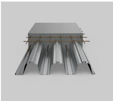
Cofraplus® 80
